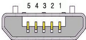
micro-USB 公头
